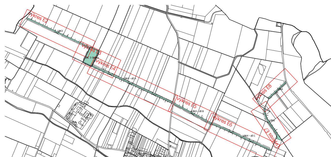
Klad listů - Schéma osazovacího plánu, M 1:25 000
